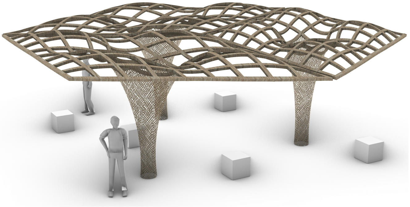
Entwurf des Demonstrationsbaus mit Stützpfeilern aus Flachsfasern und einer Dachkonstruktion aus Holz für die BUGA 2023 in Mannheim. © KIT-DDF-FibR
